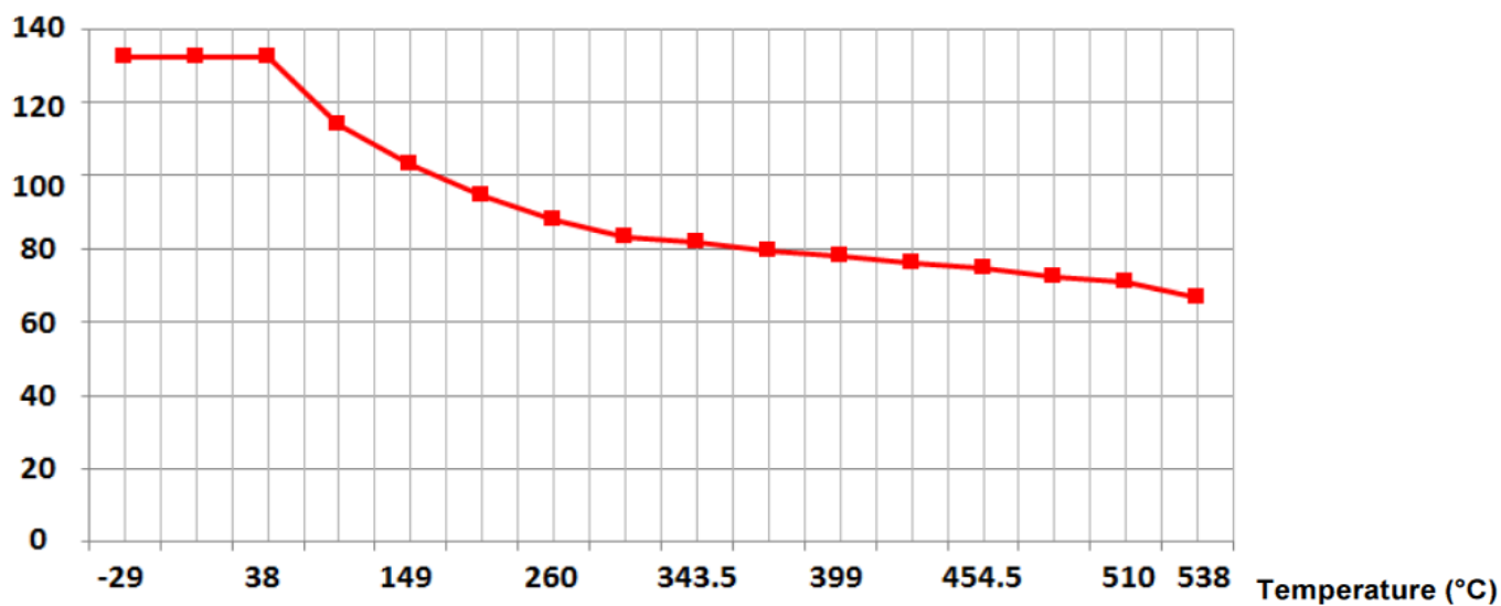
GRÁFICO PRESIÓN / TEMPERATURA - PRESSURE / TEMPERATURE GRAPH.:
