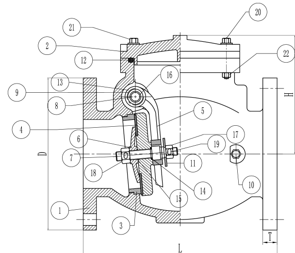
MH-XQH-300
